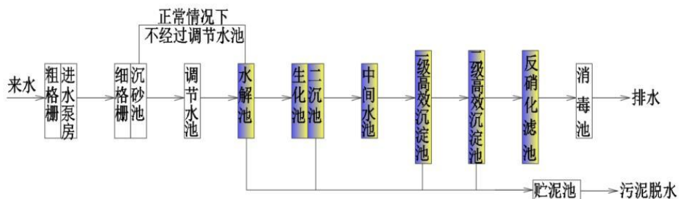
图 4-2 扩建项目污水处理工艺流程图
