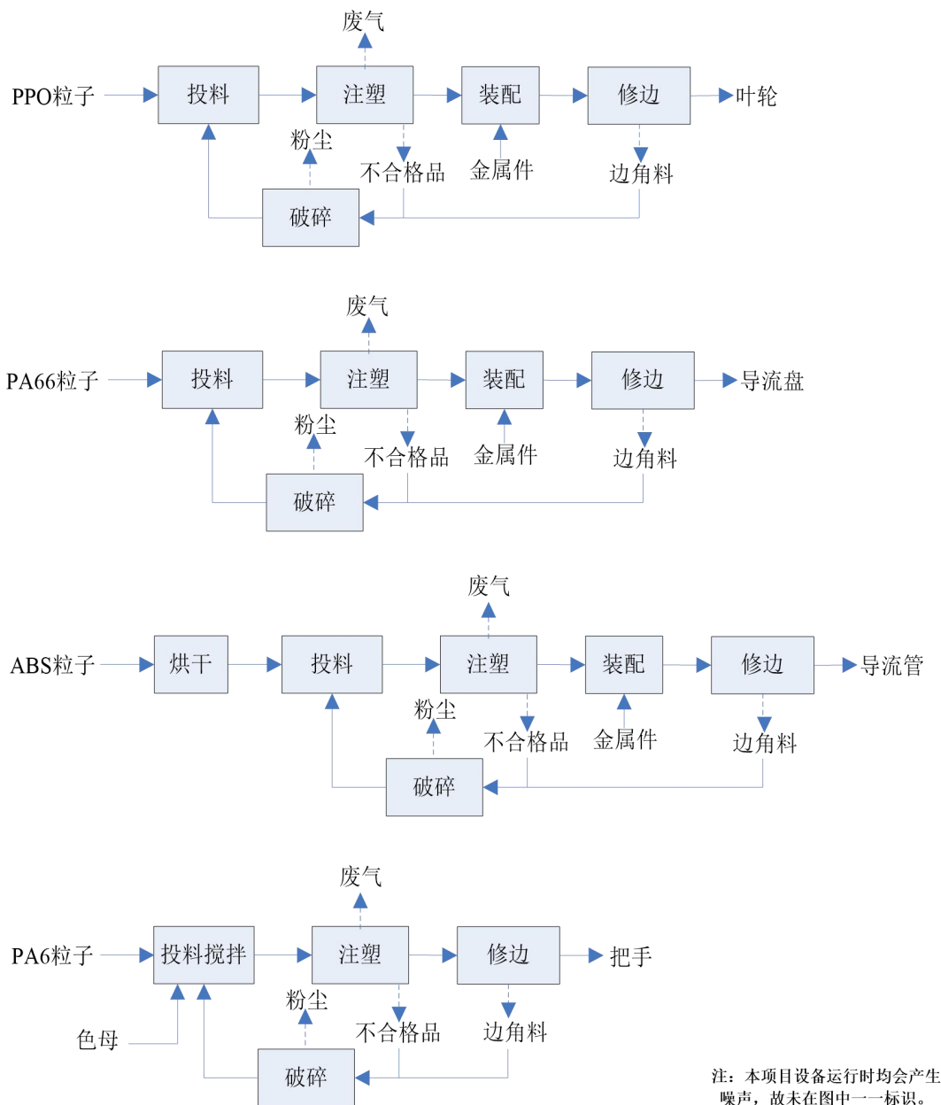
图 2-2 塑料配件生产工艺及产污流程图
