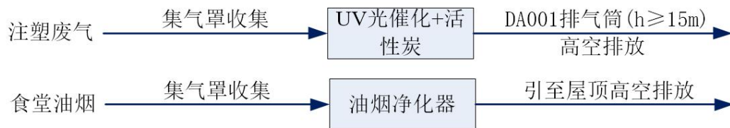
图 4-1 废气处理工艺图
