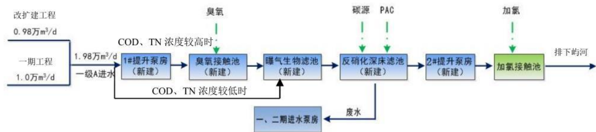
图 4-3 提标改造工程污水处理工艺流程图
