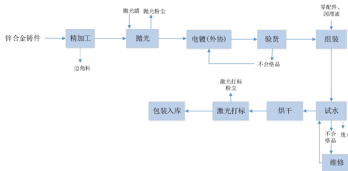
图 2-3 水龙头(锌)生产工艺及产污流程图
